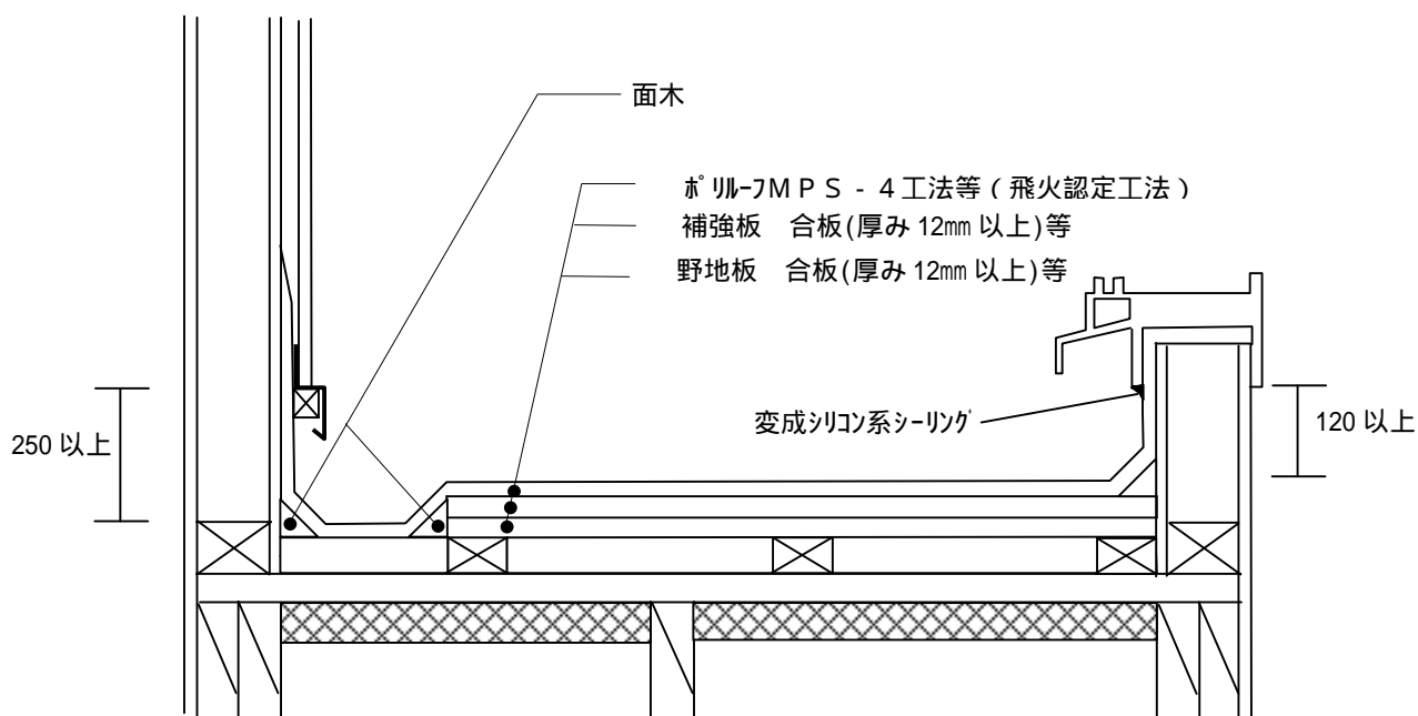
断面図 1-1
