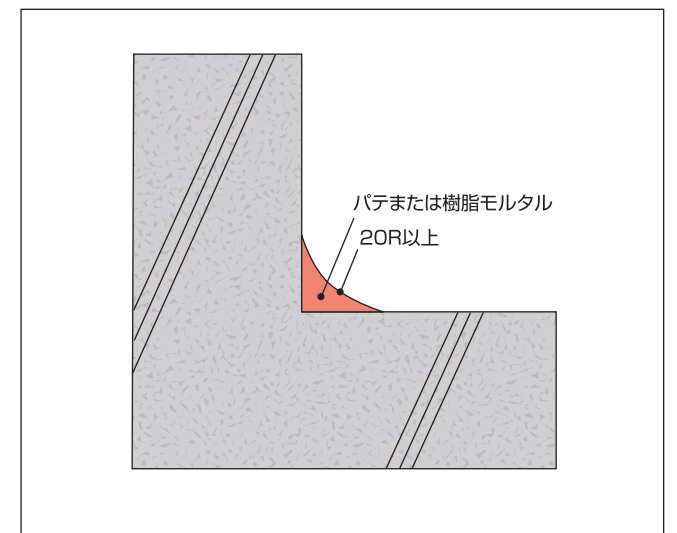
出入隅の面取り 入隅
