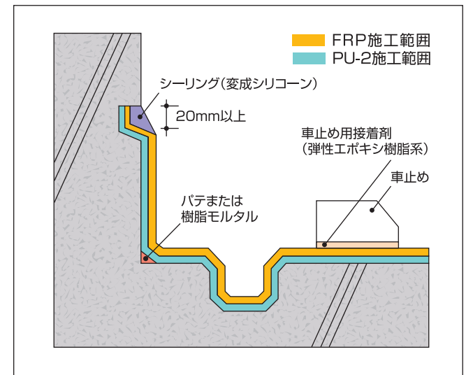
目地処理仕様
