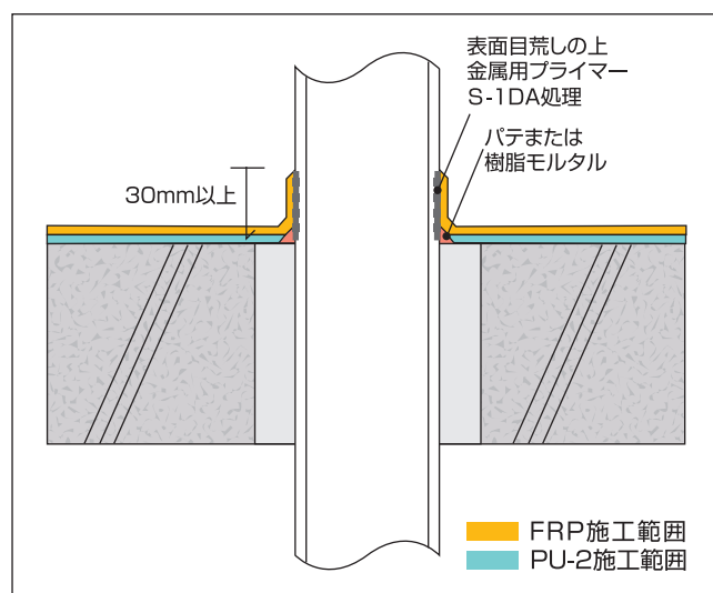
貫通パイプ
