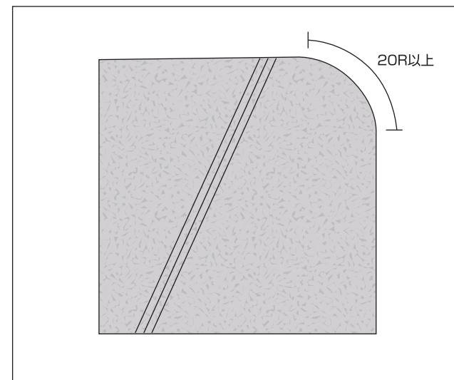
出入隅の面取り 出隅
