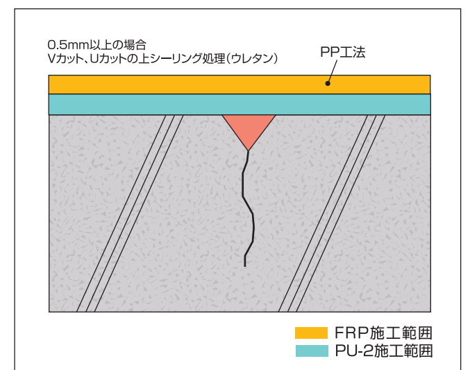
下地クラック処理2
