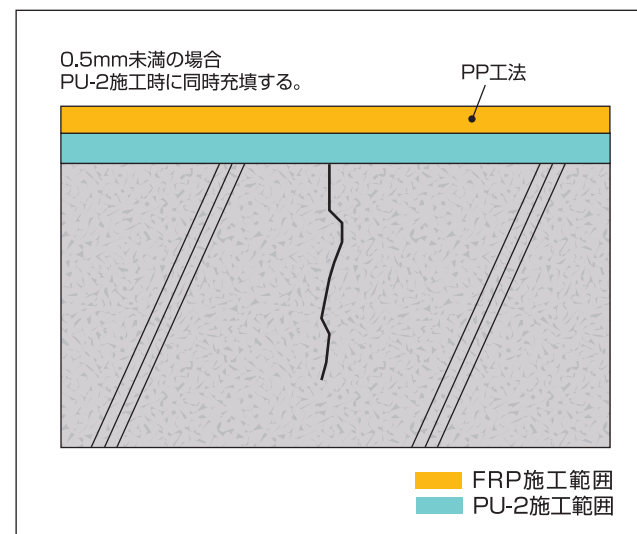
下地クラック処理1
