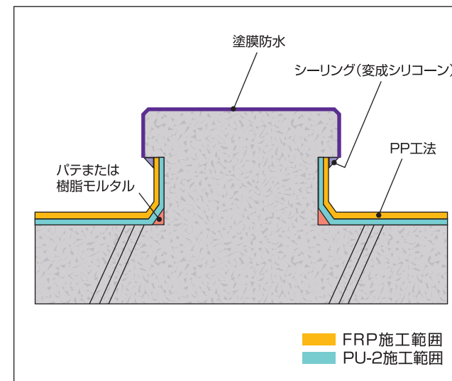
基礎架台取合部
